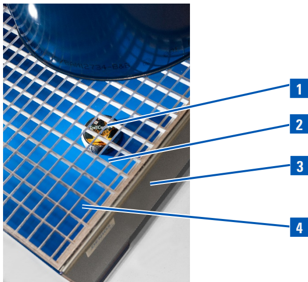
Rys. 5. SpillGuard® w wannie wychwytowej
