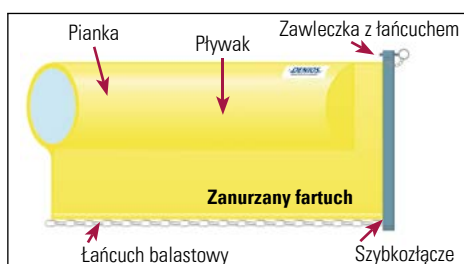
Zasada budowy bariery przeciwolejowej DENIOS
